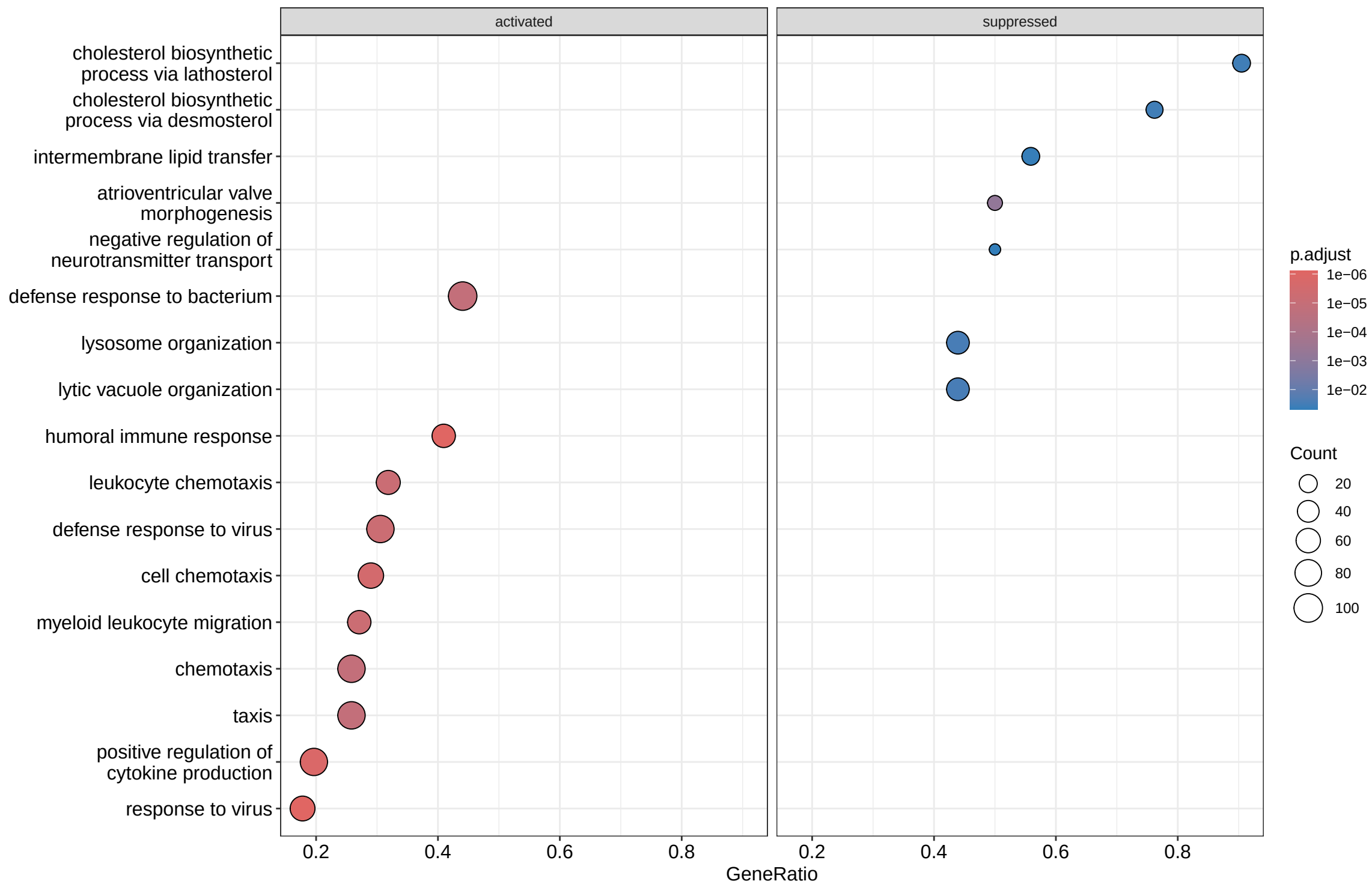
GSEA: Vias Biológicas (Ativadas vs Suprimidas em C3KO)
